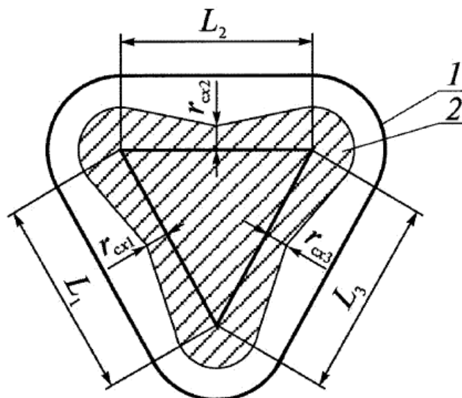
Рисунок 10. Схема зоны защиты (в плане) многократного стержневого молниеотвода: L1 , L2 , L3 - расстояния между молниеотводами; 1, 2 - границы зон защиты на уровнях соответственно земли и высоты защищаемого сооружения
