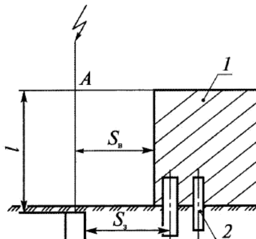
Рисунок 1. Отдельно стоящий стержневой молниеотвод: l - протяженность токопровода от точки А до заземлителя; S_в - наименьшее допустимое расстояние до защищаемого сооружения; S_з - наименьшее допустимое расстояние от заземлителя до металлических коммуникаций; 1 - защищаемое сооружение; 2 - металлические коммуникации
